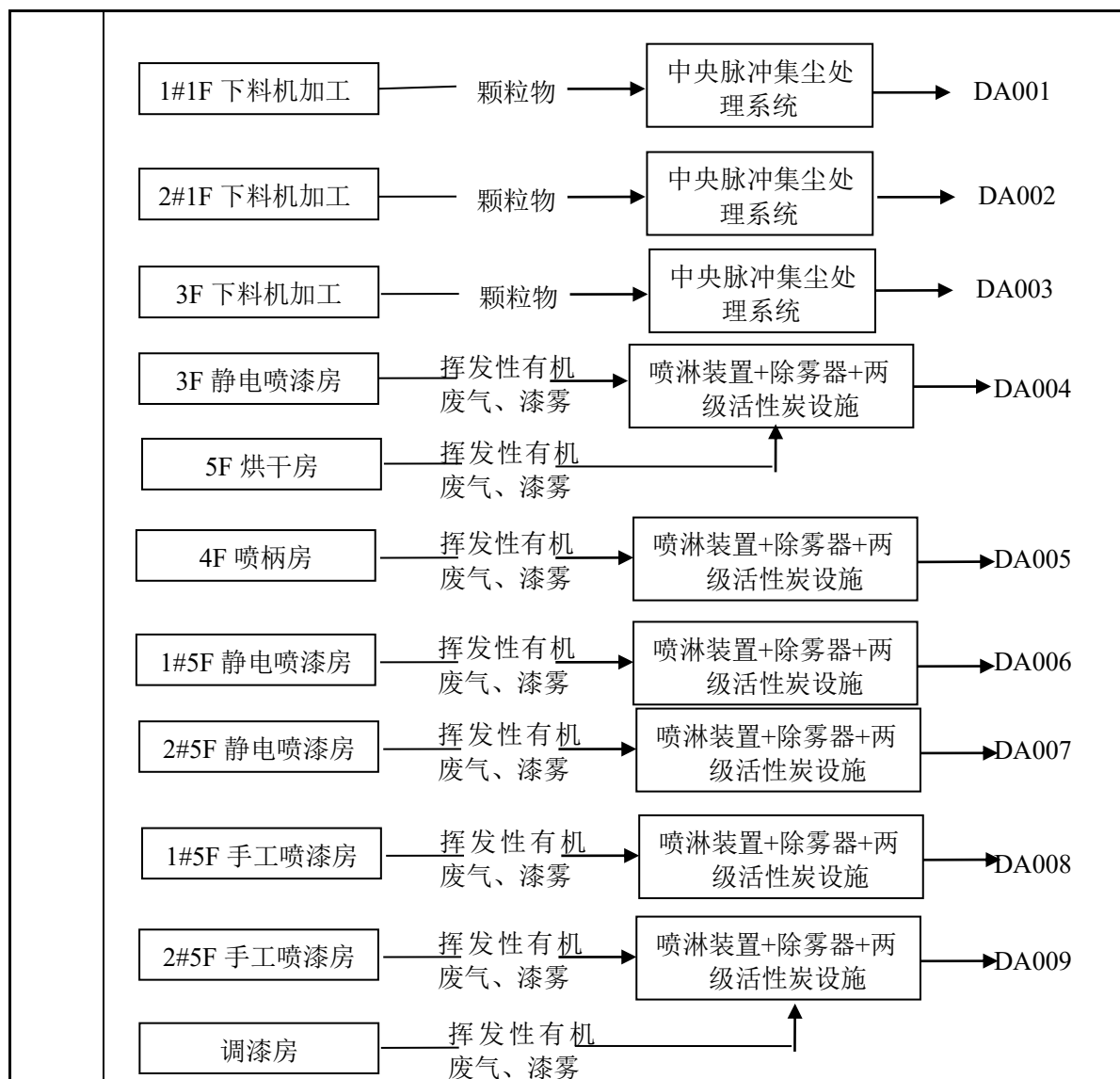
图 4-1 生产线工艺废气治理技术路线图
