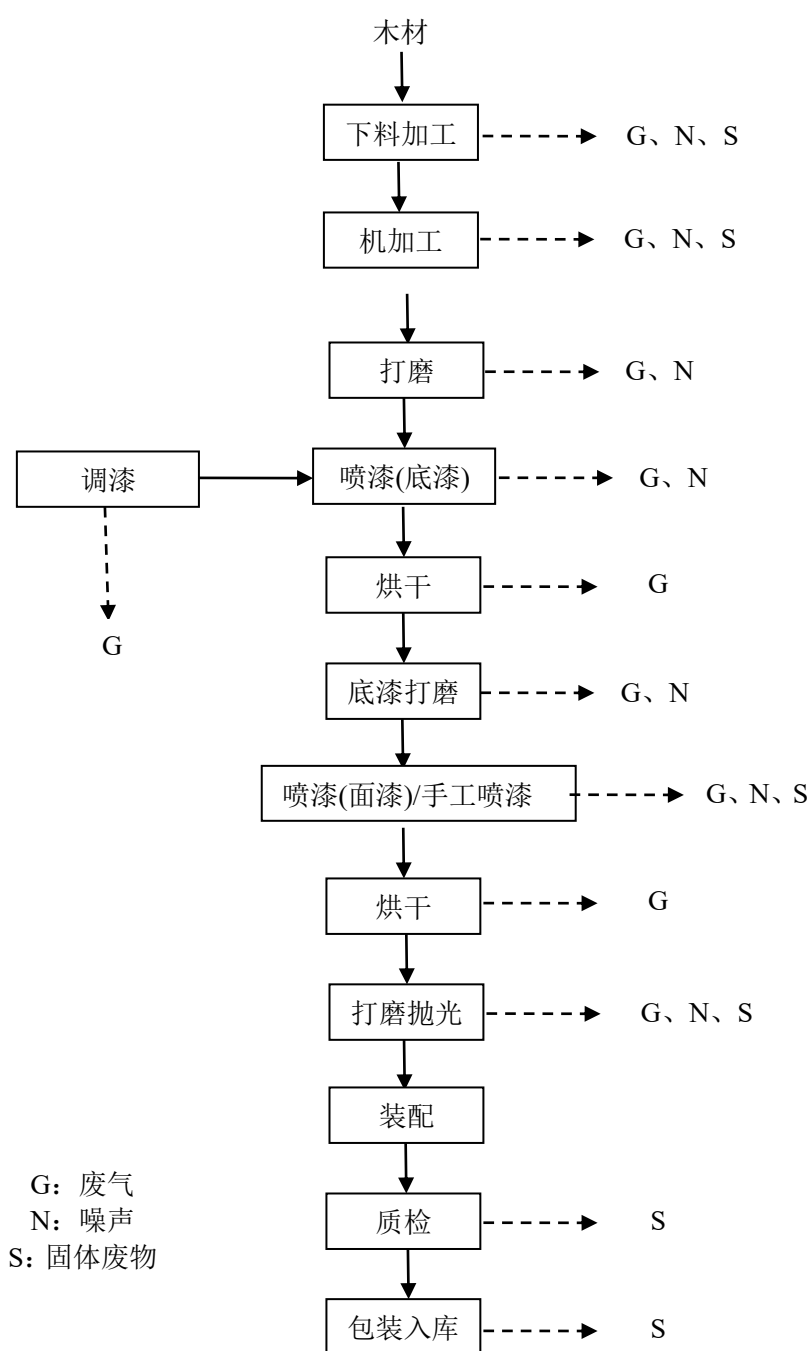
图 2-3 运营期流程及产污节点图
