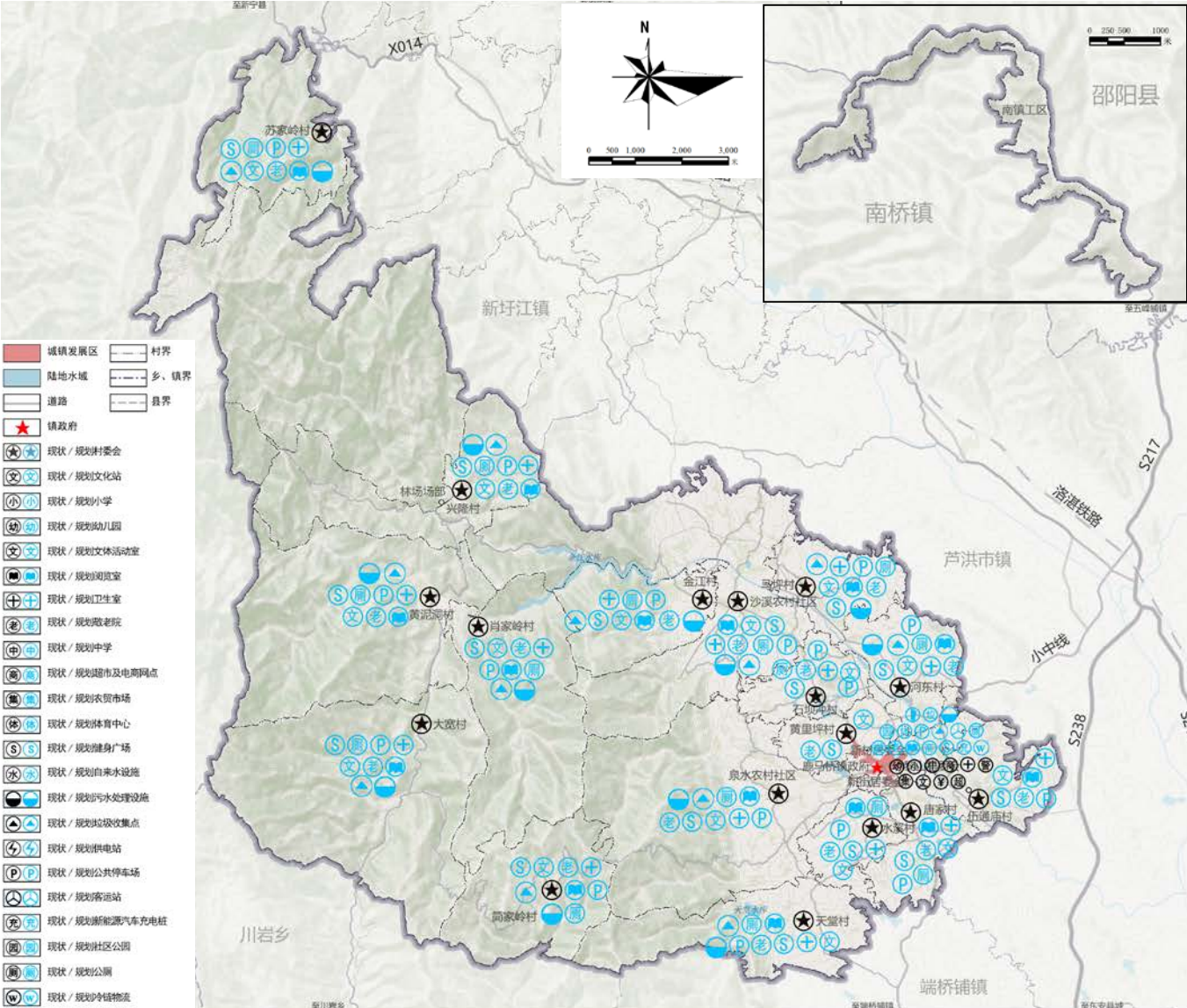
鹿马桥镇公共服务和市政基础设施规划图
