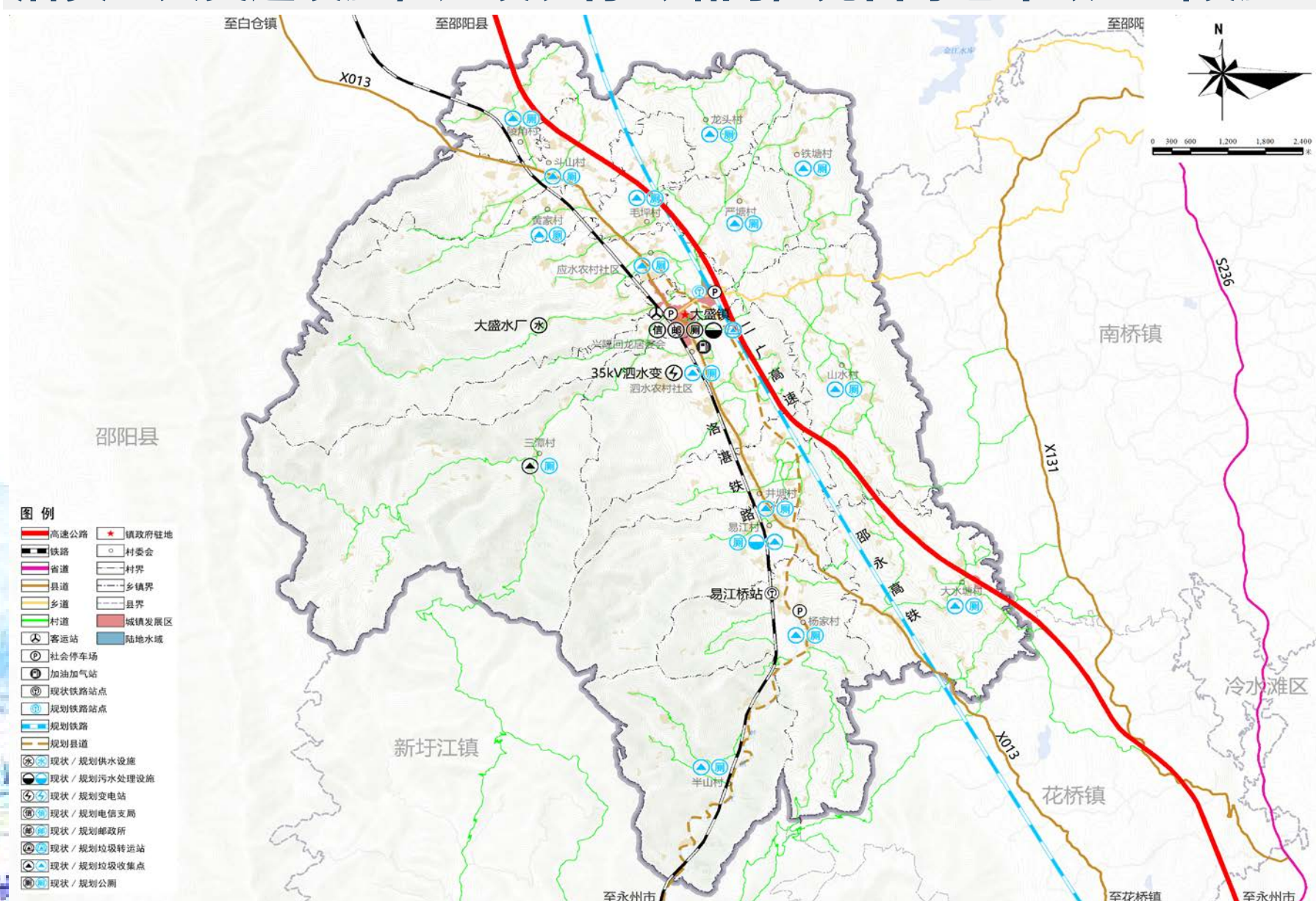
镇域综合交通与市政基础设施规划图
